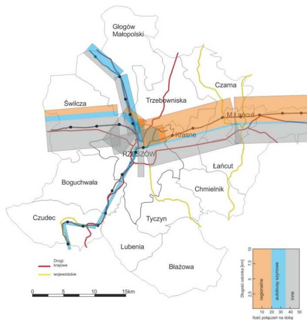
Ryc. 71. Przeciętna dobowa liczba pociągów na sieci zarządzanej przez PKP wg odcinków sieci i kategorii pociągów (styczeń-listopad 2012) w MOF Rzeszów.
