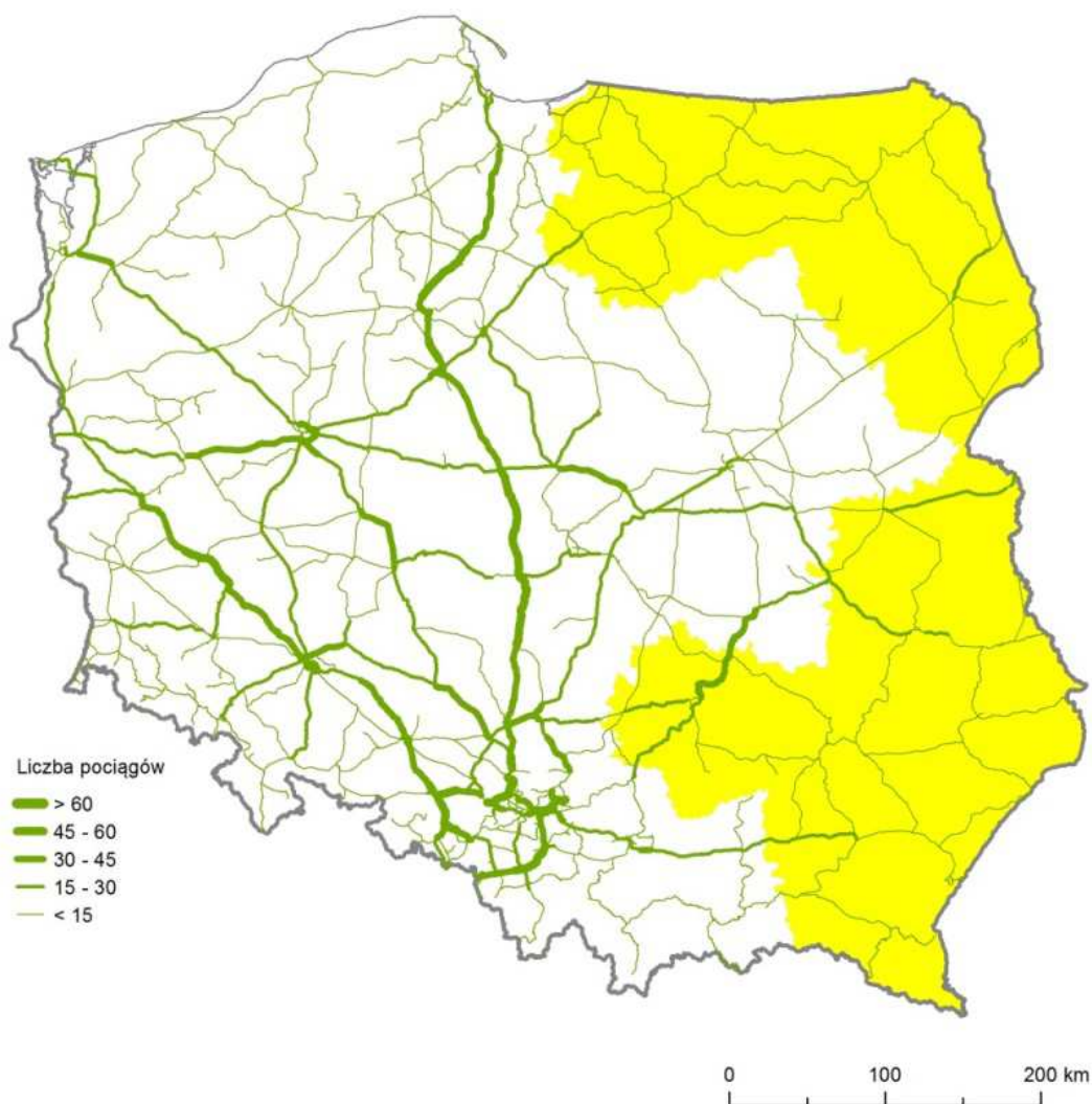
Ryc. 28. Przeciętna dobowa liczba pociągów towarowych na sieci zarządzanej przez PKP PLK w 2010 r.
