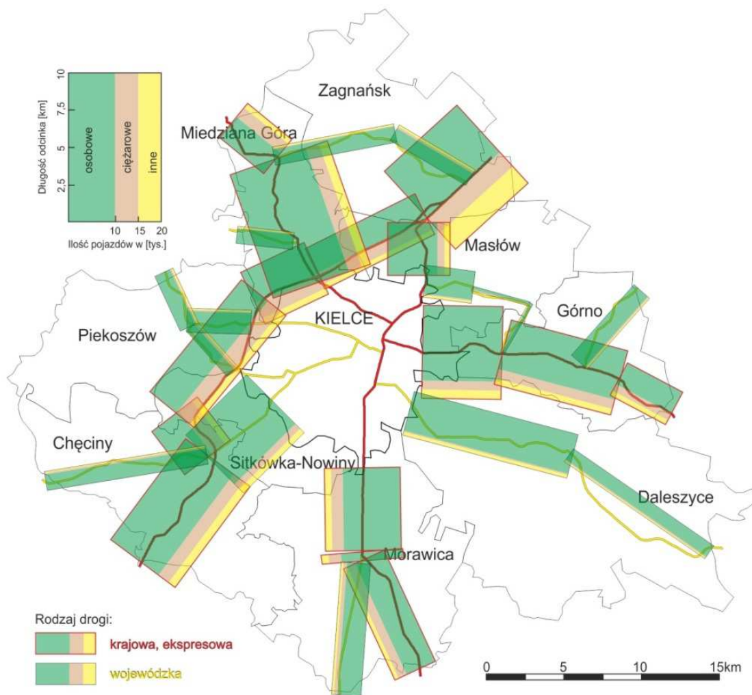
Ryc. 84. Natężenie ruchu na sieci zamiejskich dróg krajowych i wojewódzkich w 2010 r. według kategorii pojazdów na obszarze MOF Kielce.
