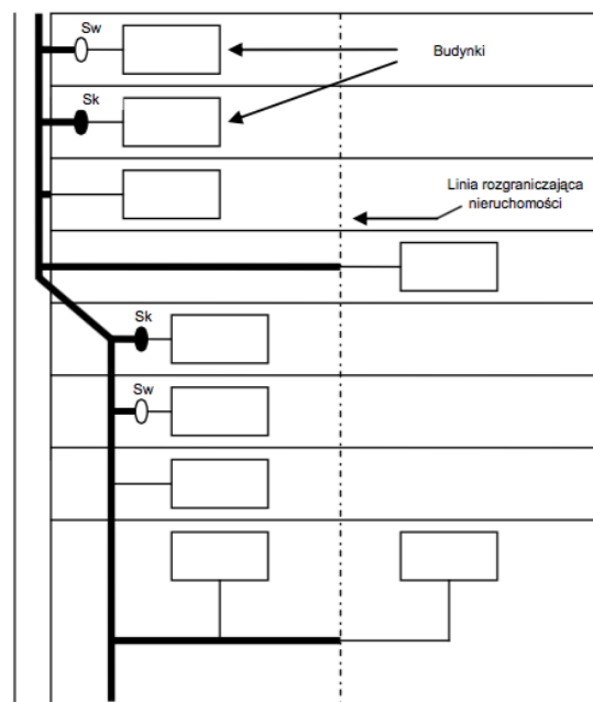
Rysunek 1. Kanalizacja grawitacyjna i wodociągi Pogrubione odcinki wodociągu stanowią element kwalifikowalny.
